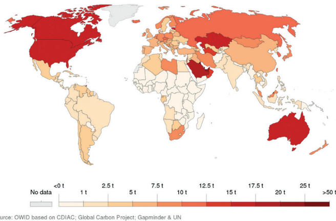
Figure 12.3 : Émissions de CO 2 par habitant et par an dans le monde en 2017. Source : Our World in Data https://fr.wikipedia.org/wiki/Fichier:CO2_emissions_per_capita,_2017_(Our_World_in_Data).svg .
