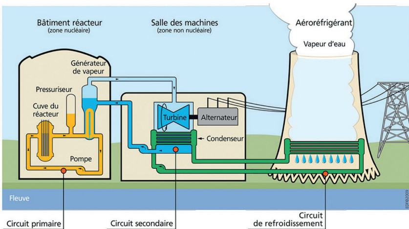
Figure 11.25 : Schéma de principe d'une centrale nucléaire avec aérorefrigérant. Source : IRSN (Institut de Radioprotection et de Sûreté Nucléaire) EDF@2009
